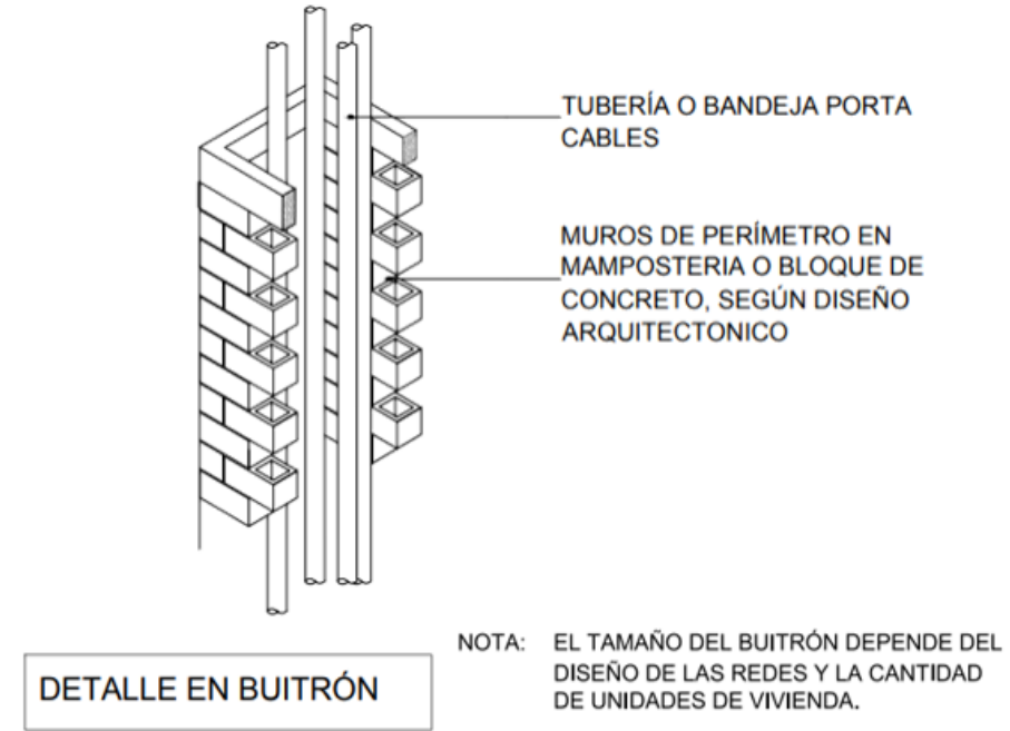
Gráfica 11. Detalle del Buitrón
