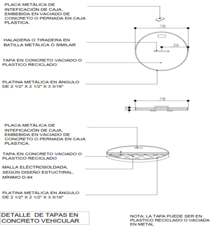
Gráfica 8. Detalle de construcción de la tapa circular
