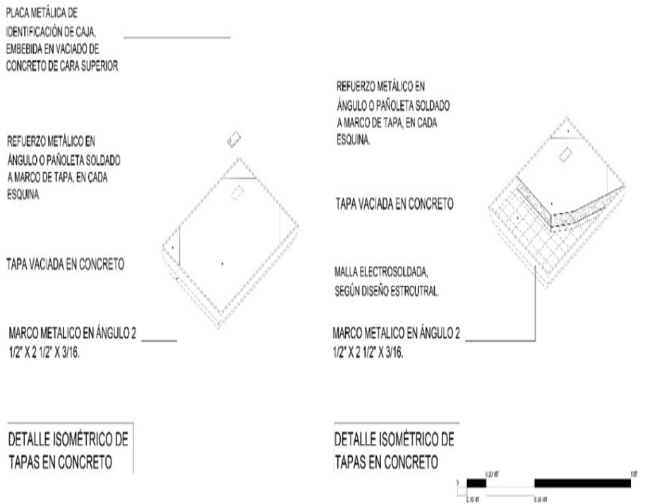
Gráfica 7. Detalle de construcción de la tapa
