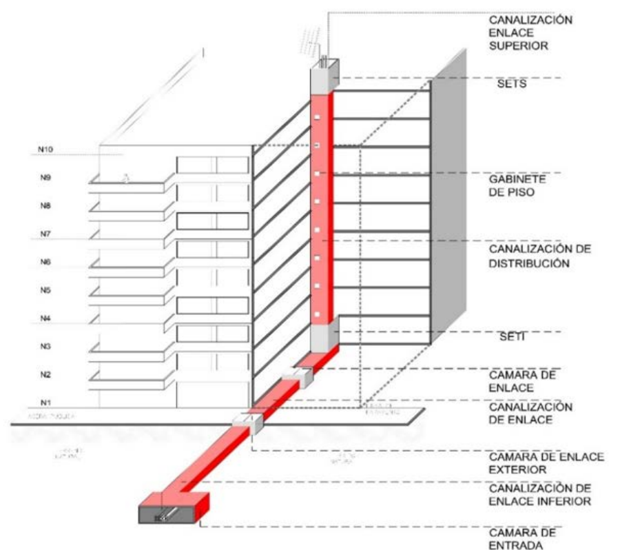
Gráfica 3. Infraestructura Soporte
