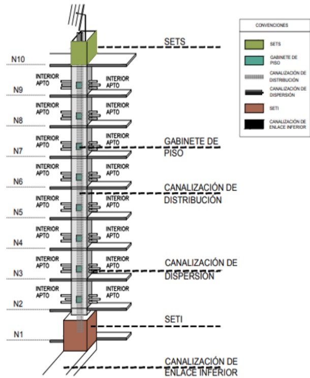
Gráfica 10. Esquema de canalización de distribución en edificios de varios pisos
