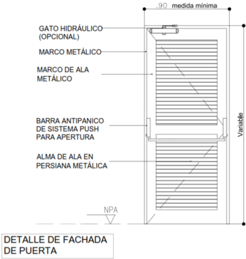
Gráfica 9. Detalle de la puerta
