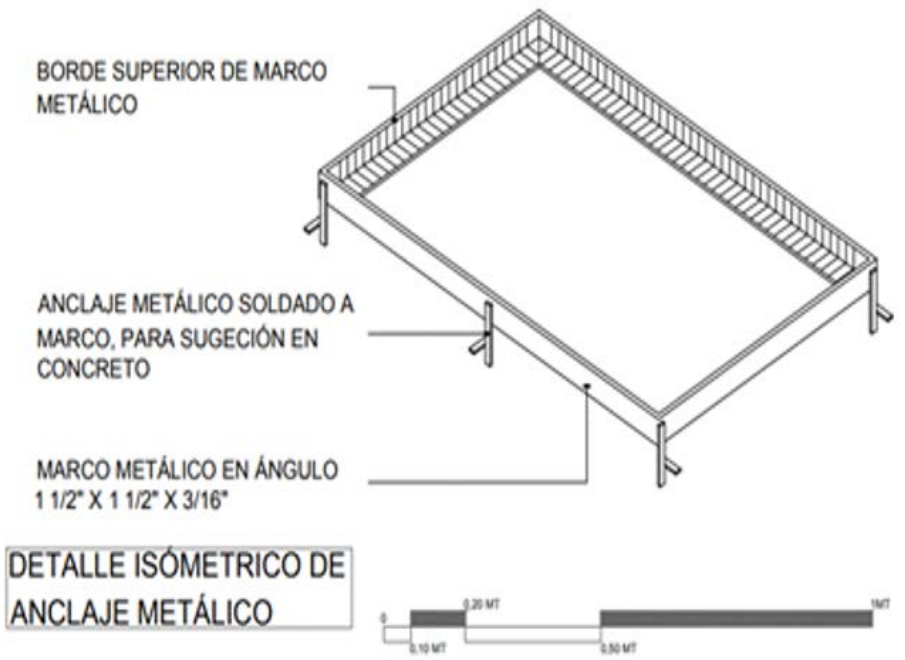
Gráfica 6. Anclaje metálico
